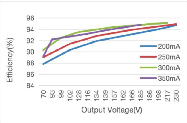
Зависимость КПД от выходного напряжения
